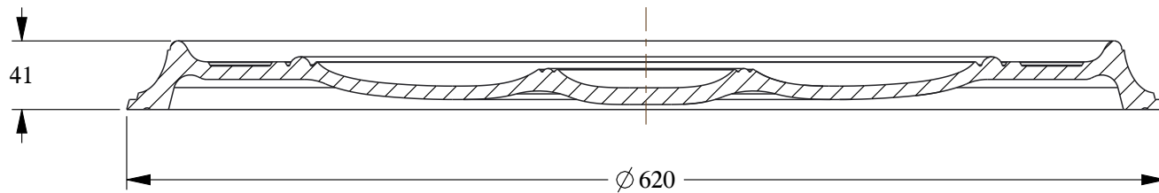
SECTION A-A
